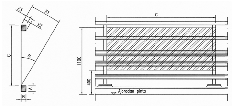
Kuva 4. Läpinäkyvyyden laskentaperiaate katsottaessa kaidetta päältä (vas.) ja läpinäkyvyyden laskenta-alue (oik.).
